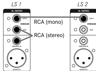
Abb. 2: Stereo Link
