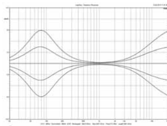
fig. 10: Room EQs
