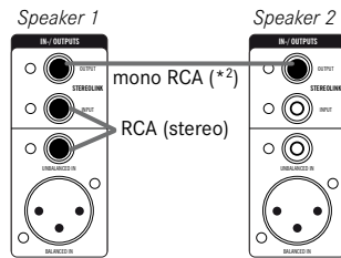
fig. 2: Stereo Link
