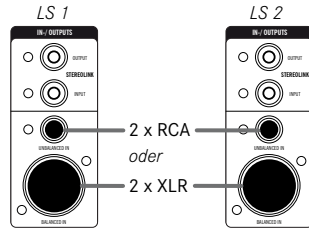
Abb. 1: ‚normaler‘ Anschluss
