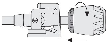
Abb. 5: Gegengewicht montieren
